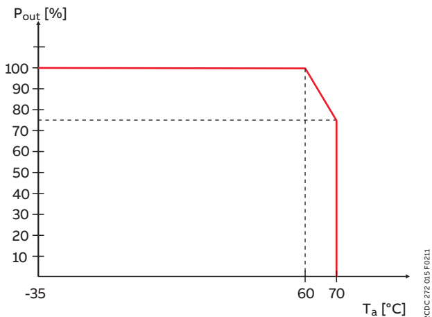
CP-E 12/10.0, CP-E 24/5.0
